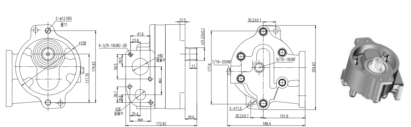
2P9239 Dimensions
